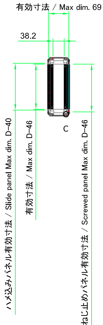
ナットレール / Nut rail
